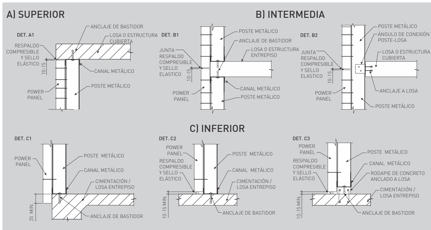
Fig. 3 Conexión de Bastidores a Estructura principal.
