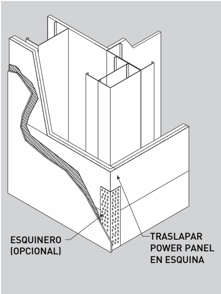
Fig. 20 Detalle de esquina.
