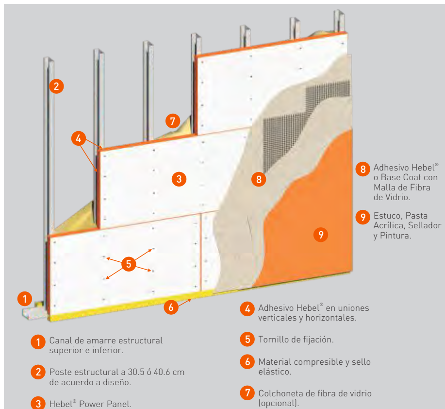
Fig. 22 Muro Exterior
